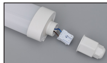
Branchements électriques rapides
