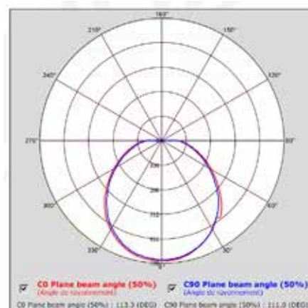
COURBE PHOTOMÉTRIQUE :
